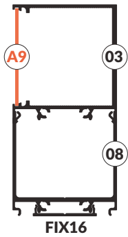
Variante 32 - seitliche Wandversion FIX16-08-03-A9 variant 32 - wall side FIX16-08-03-A9
