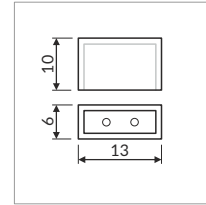
Endkappe für die Silikonhülle für LED Streifen mit 8 mm ending for silicone housing for 8 mm LED strip
